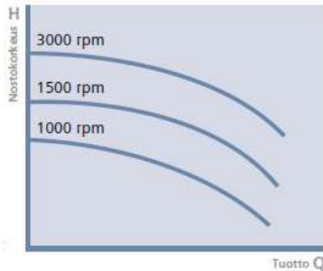
QH-käyrä
